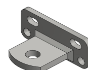
Beslag med laske 691271 inkl. rørbøjle for 70 x 70 stolpe 691271-01 inkl. bolte M10x40
